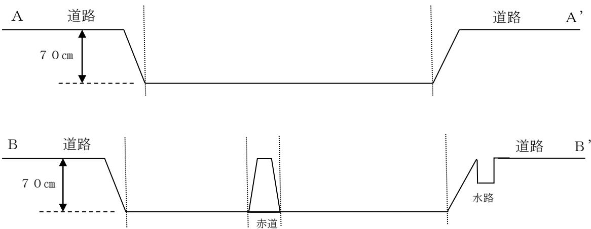
(現況断面図)
