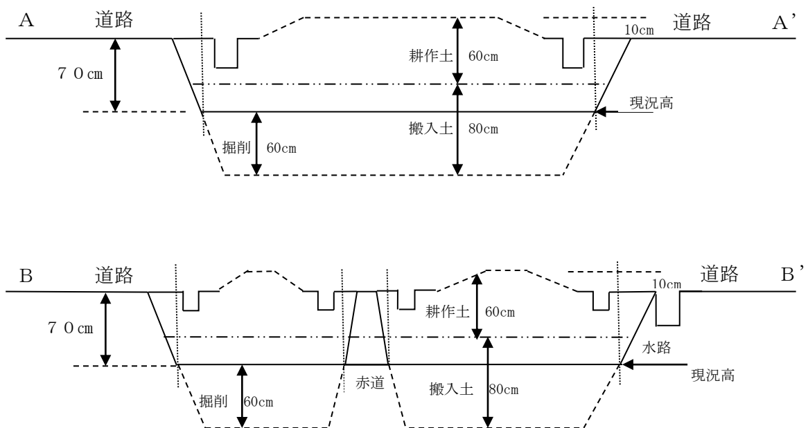
(改良断面図)
